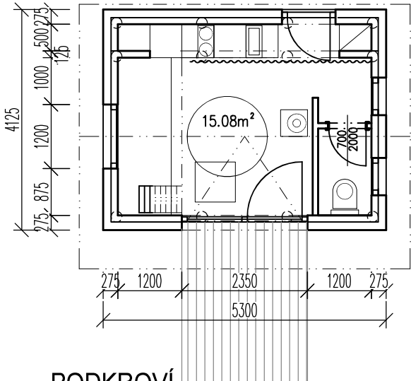
PODKROVÍ
