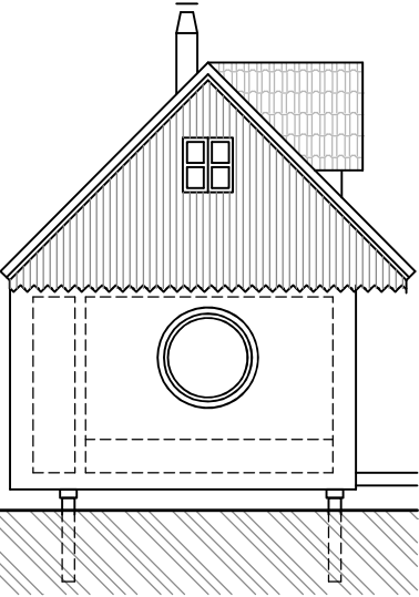
POHLED JIH
