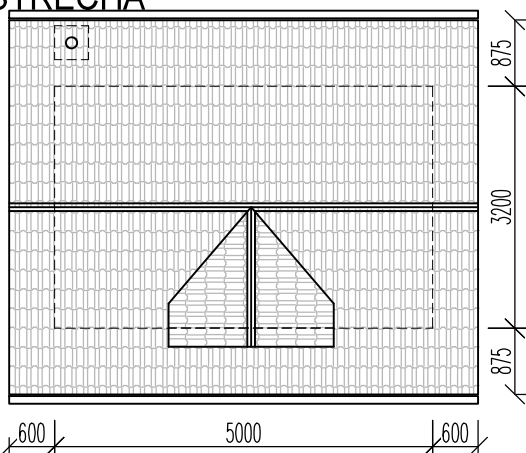
PODKROVÍ
