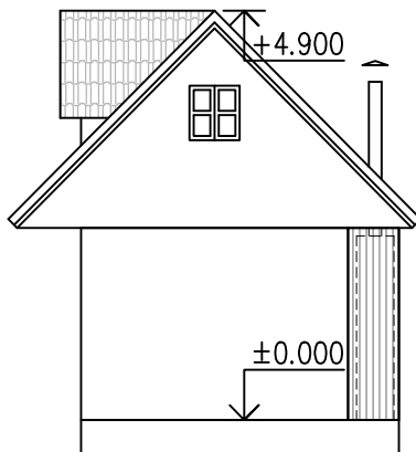
POHLED ZÁPAD
