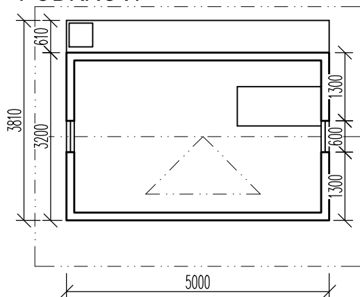
1.NP
