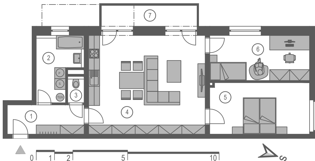
PŮDORYS BYTU
