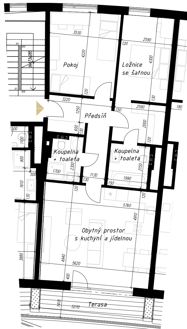
PŮDORYS JEDNOTKY / M 1:100
