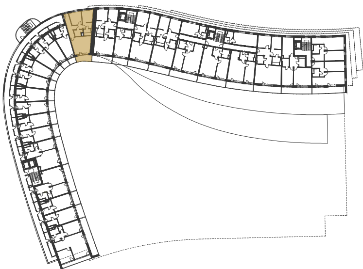
SCHEMA UMÍSTĚNÍ JEDNOTKY NA PODLAŽÍ / M 1:1000
