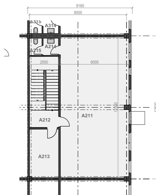
PŮDORYS 2.NP
