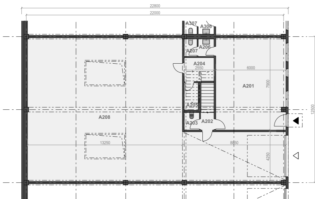
PŮDORYS 1.NP
