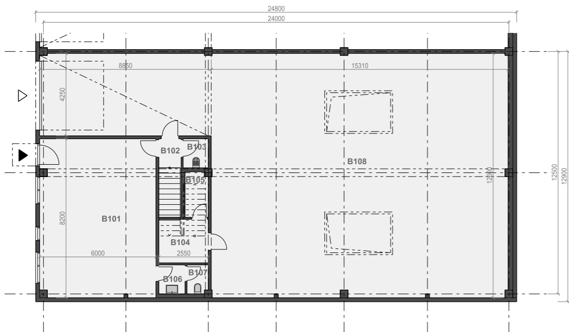
PŮDORYS 1.NP
