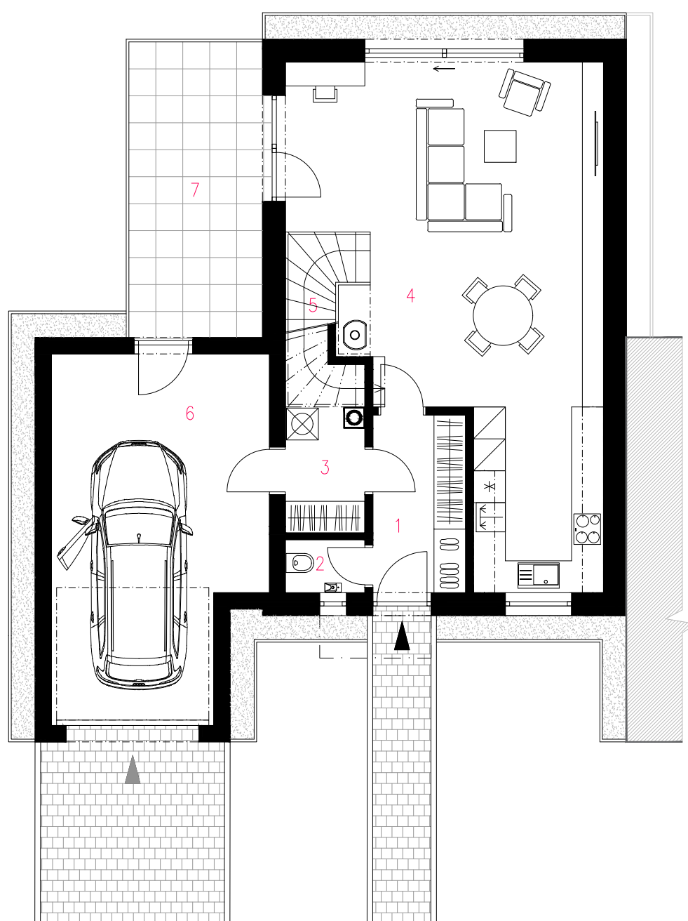
Půdorys 1.np
