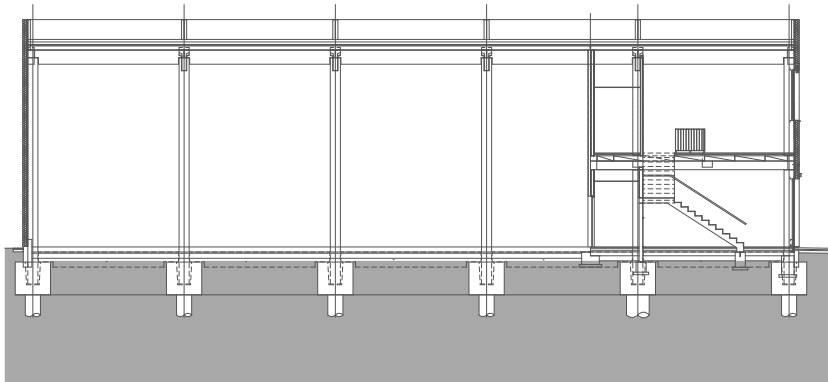
Podélný řez
