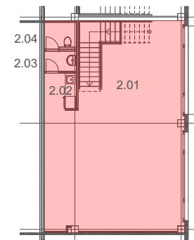
Půdorys 2.NP
