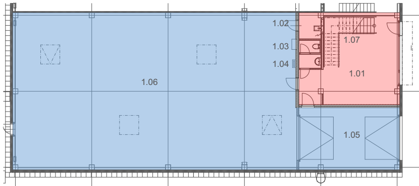
Půdorys 1.NP
