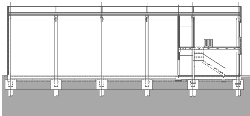
Podélný řez
