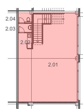
Půdorys 2.NP
