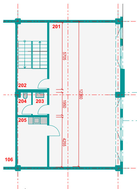
PŮDORYS 2NP
