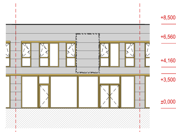
POHLED JIHOVÝVODNÍ
