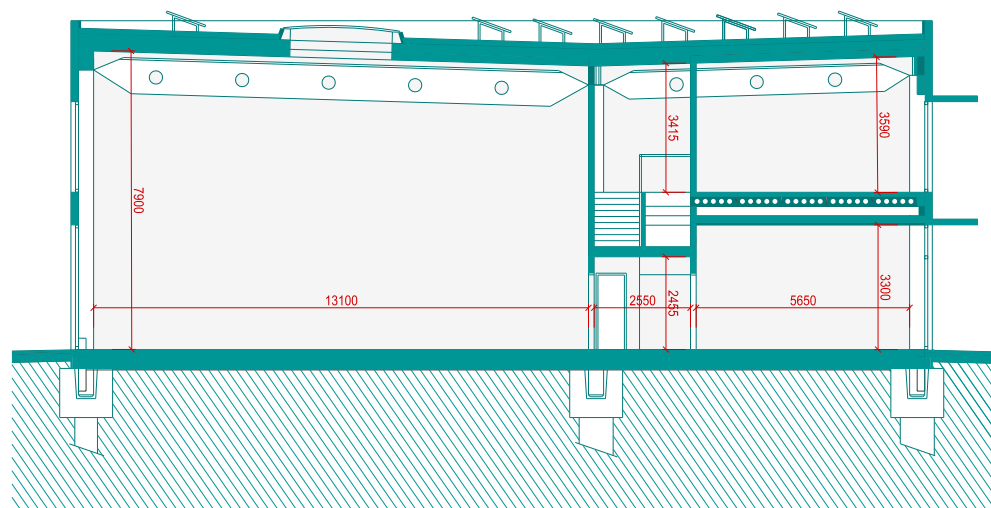
PŘÍČNÝ ŘEZ
