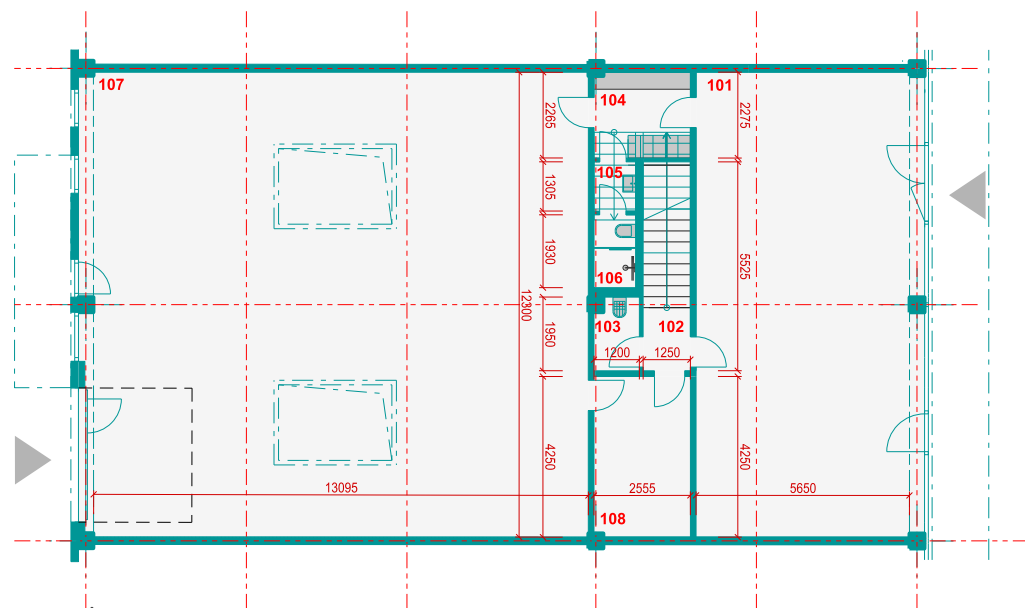
PŮDORYS 1NP
