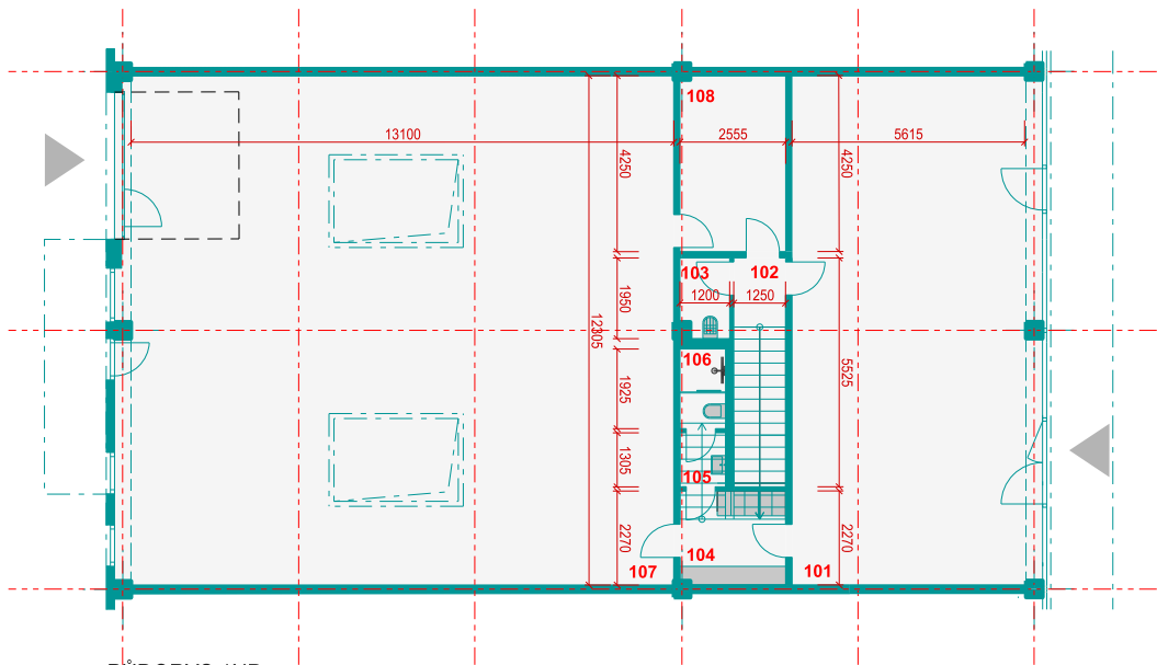
PŮDORYS 1NP
