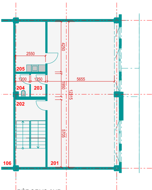
PŮDORYS 2NP
