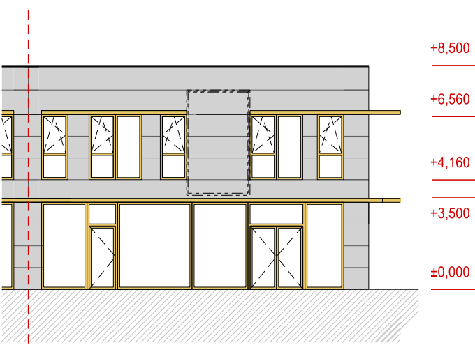
POHLED JIHOVÝVODNÍ
