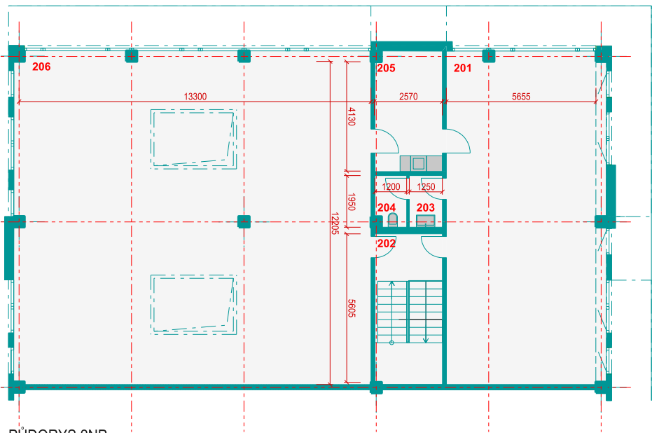
PŮDORYS 2NP
