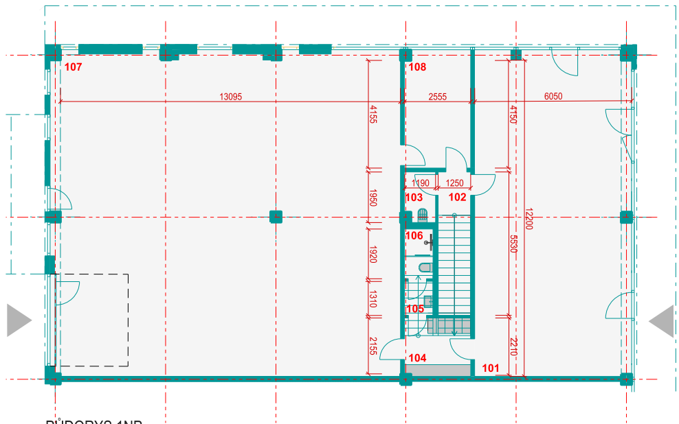
PŮDORYS 1NP
