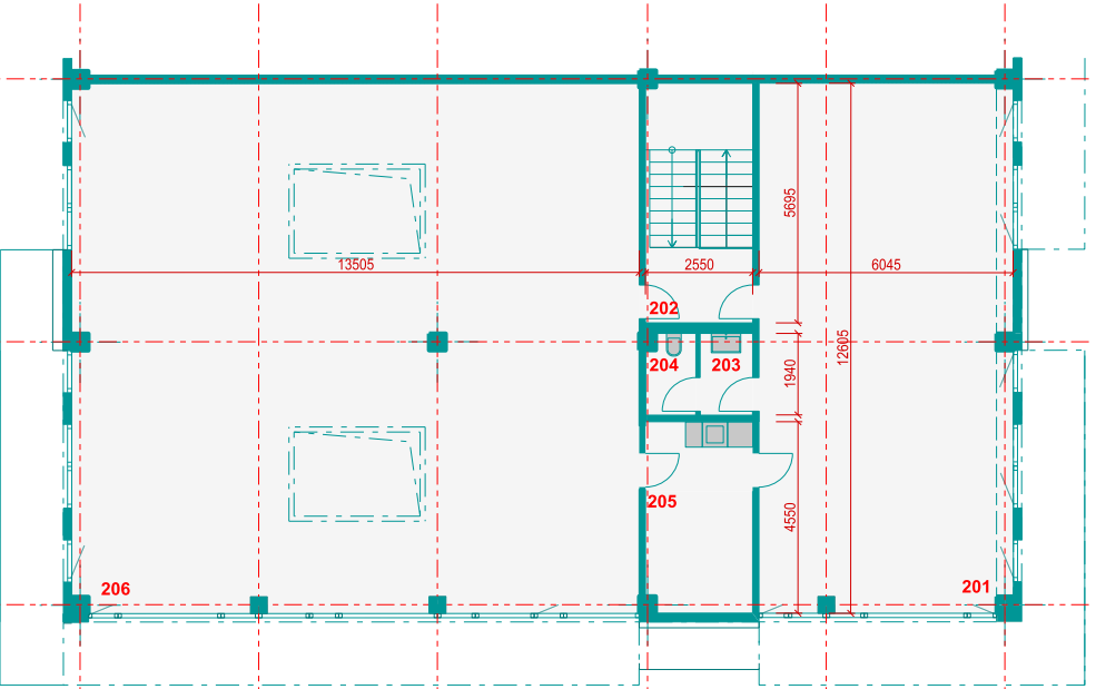
PŮDORYS 2NP
