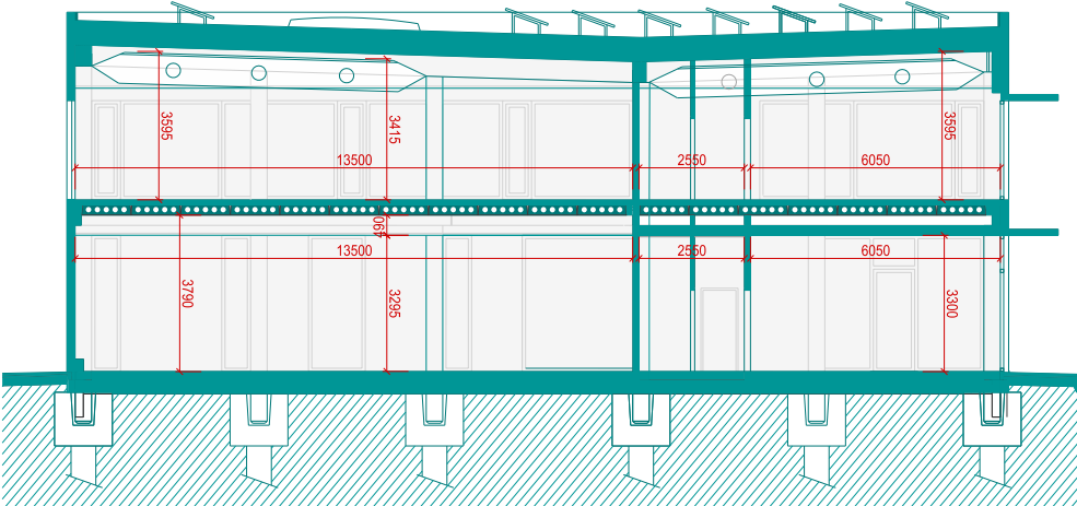
PŘÍČNÝ ŘEZ
