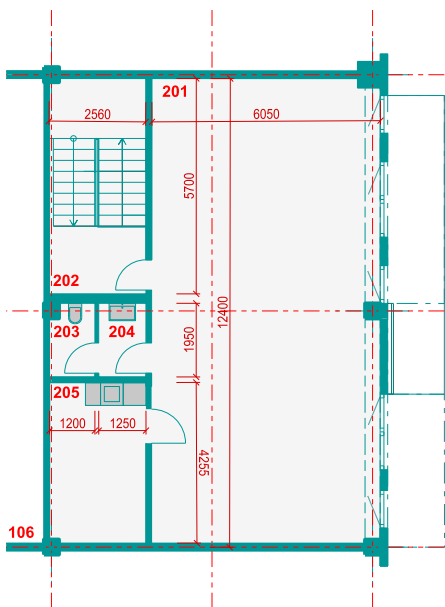
PŮDORYS 2NP
