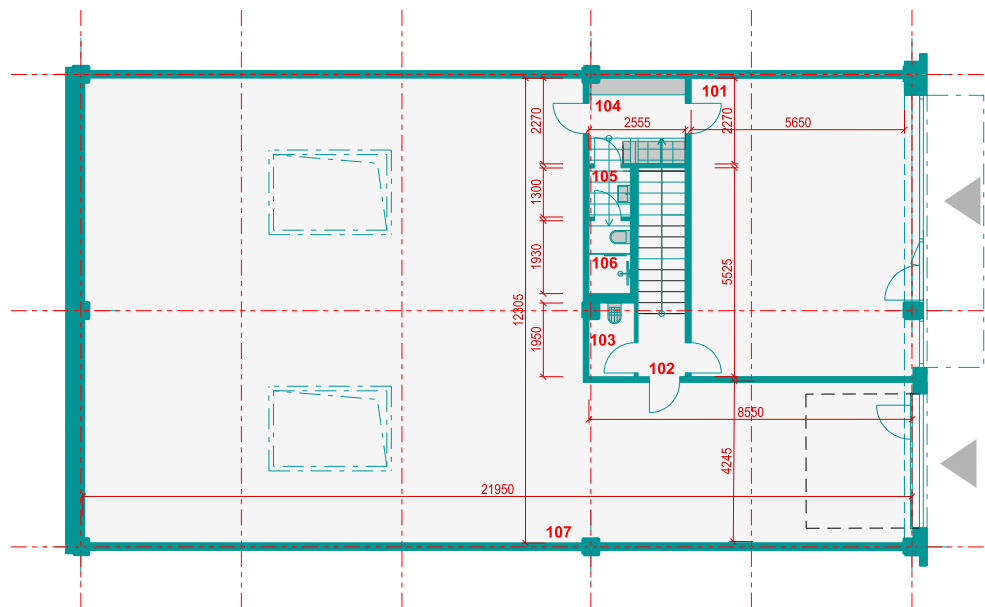
PŮDORYS 1NP
