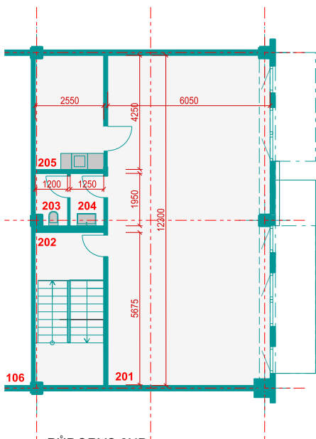
PŮDORYS 2NP
