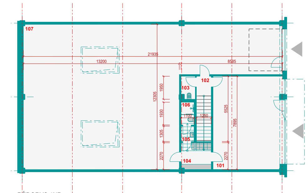
PŮDORYS 1NP
