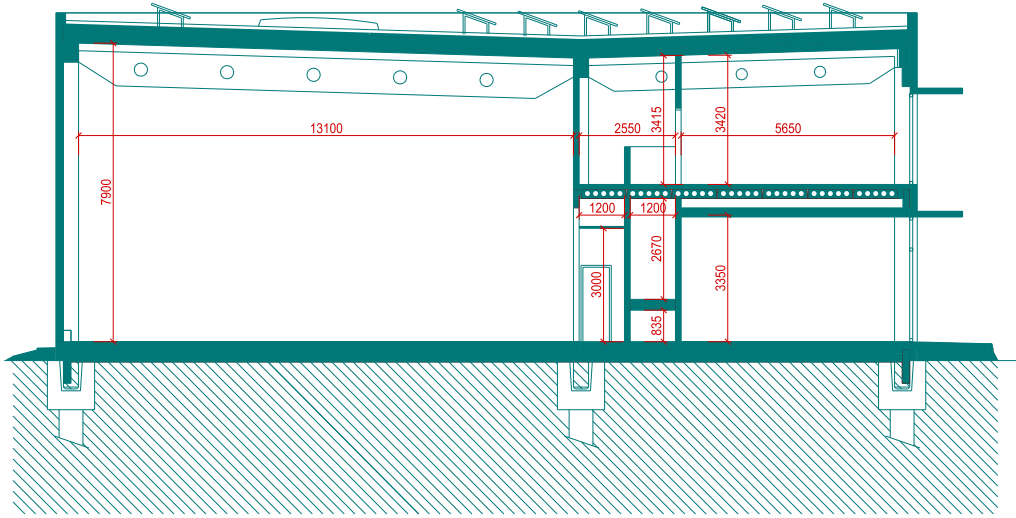
PŘÍČNÝ ŘEZ
