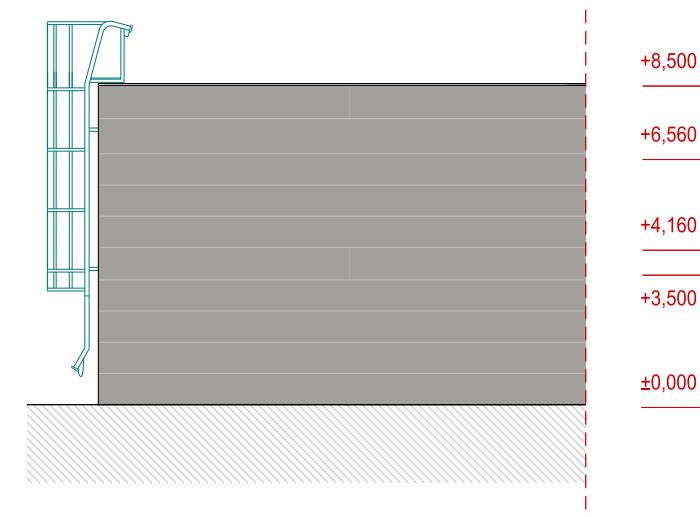
POHLED SEVEROZÁPADNÍ
