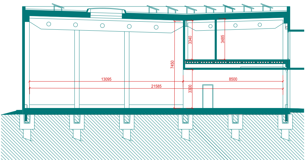
PŘÍČNÝ ŘEZ
