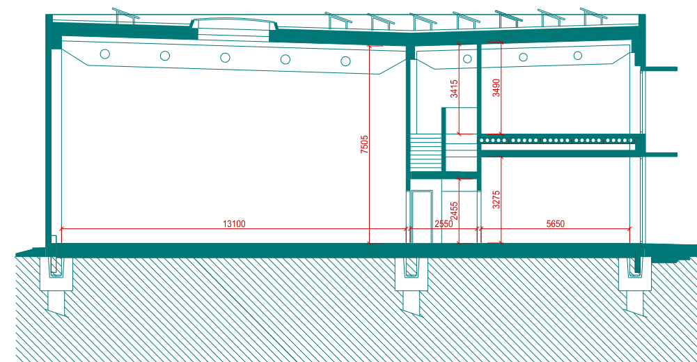
PŘÍČNÝ ŘEZ
