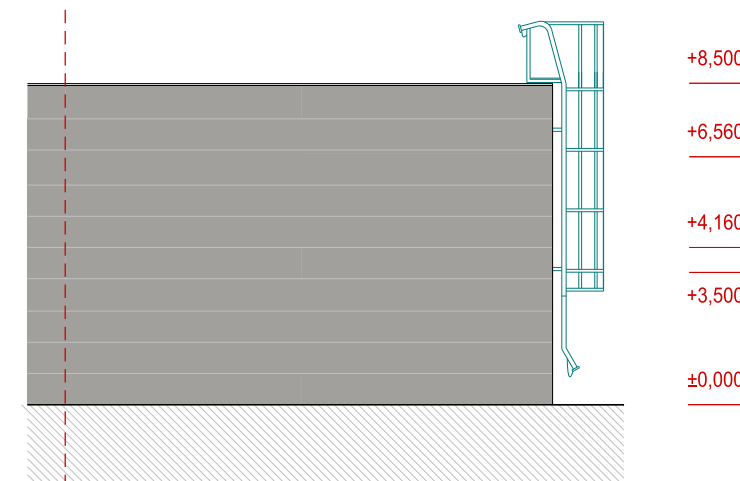
POHLED SEVEROZÁPADNÍ
