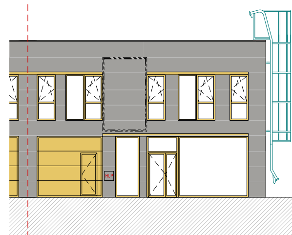
POHLED JIHOVÝVHODNÍ
