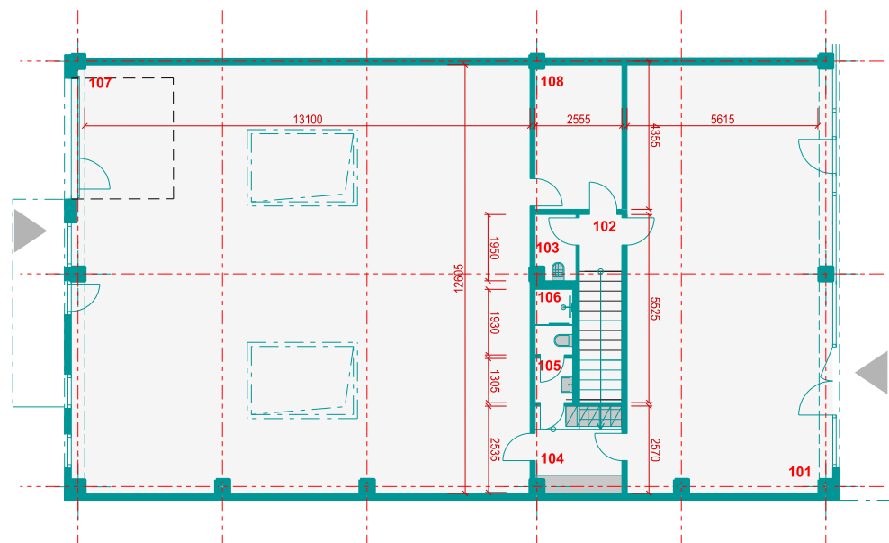
PŮDORYS 1NP
