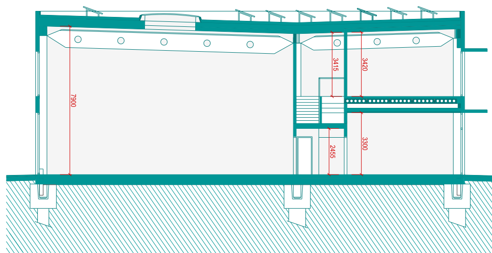
PŘÍČNÝ ŘEZ
