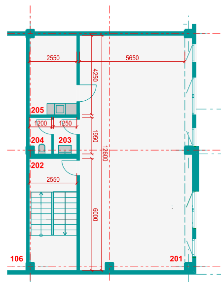
PŮDORYS 2NP
