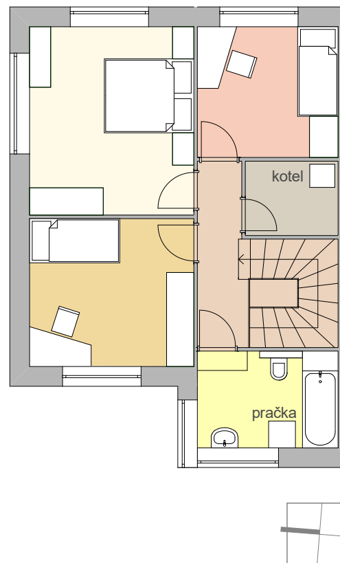
PŮDORYS 2.NP
